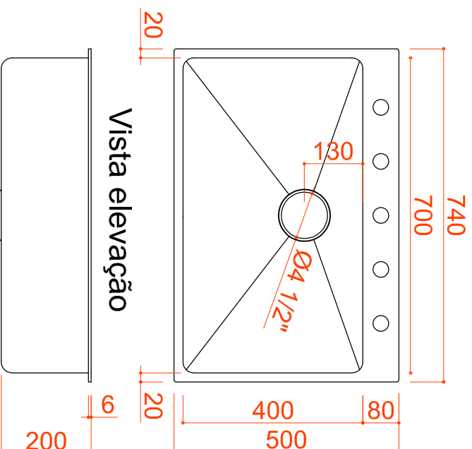
Vista planta
