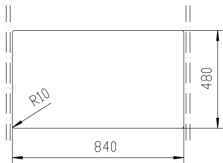
Ausschnitt übergreifend M 1:20
